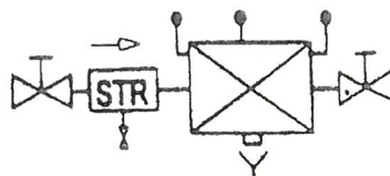
Bild 3 – Sicherungseinrichtung BA
